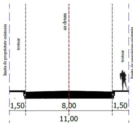
A-A' - BULEVARDUL TRAIAN (profil existent conform ridicare topografică) SC 1:200
